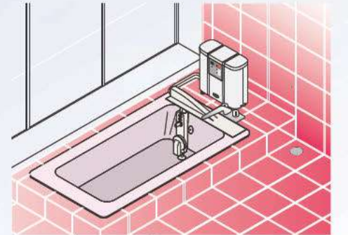
スタンダードタイプ ゆとりある浴室床面や棚面を利用してレイアウトします。
